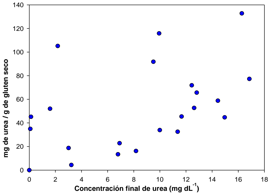
Figura 10. Isotherma de adsorción de urea en agua destilada a 25 °C.
