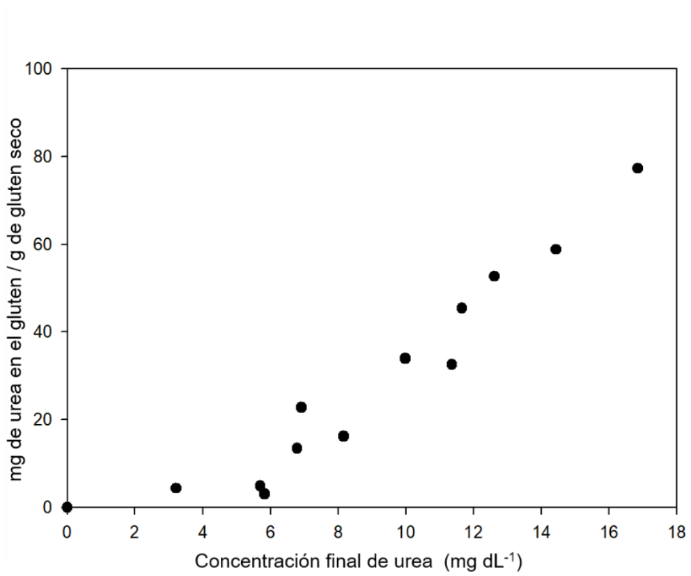
Figura 11. Isotherma de adsorción de urea de gluten seco en agua destilada a 25 °C.
